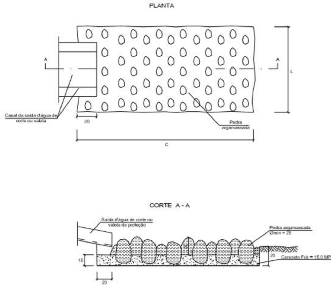
DEN - DISSIPADOR DE ENERGIA PARA SAÍDA D'ÁGUA E VALETA DE PROTEÇÃO DE CORTE
