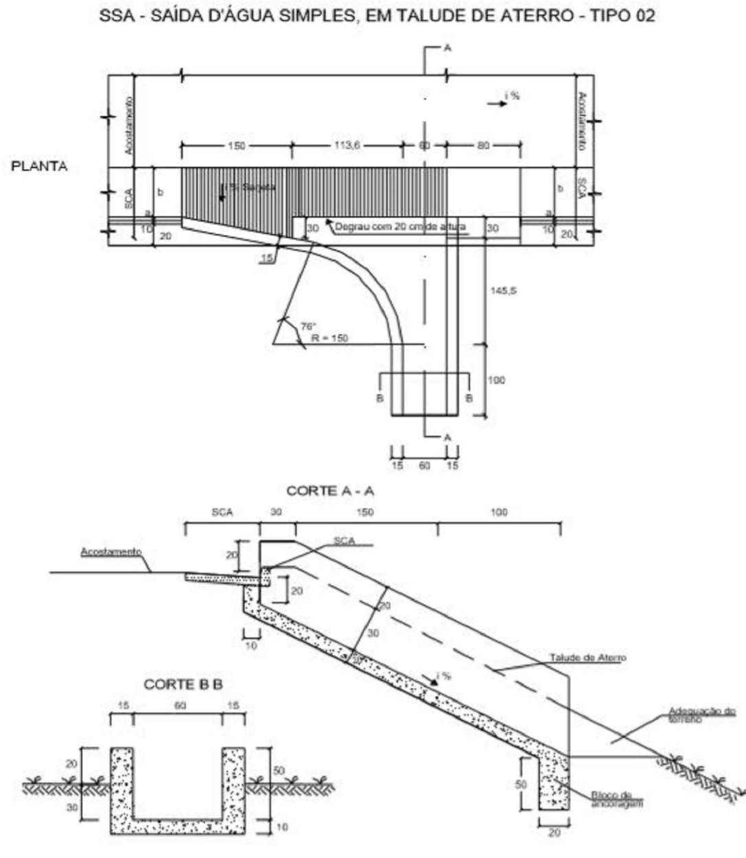
SAÍDAS D'ÁGUA SIMPLES E DUPLA - SSA-02
