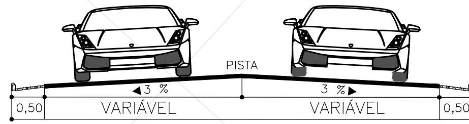
SEÇÃO TIPO – RUAS S/ ESCALA
