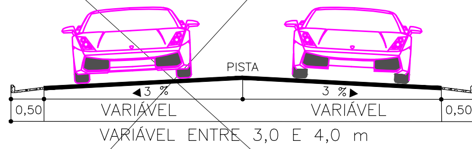
SEÇÃO TIPO - RUAS S/ ESCALA
