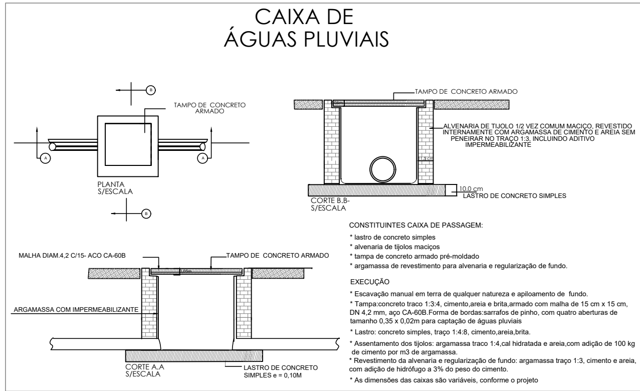
Detalhe SAN-4 Escala 1:25
