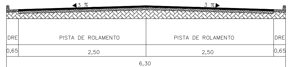
SEÇÃO TIPO - 6,30 m PAVIMENTO CBUQ SEM ESCALA
