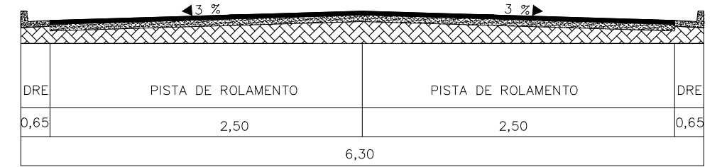
SEÇÃO TIPO - 6,30 m PAVIMENTO CBUQ SEM ESCALA
